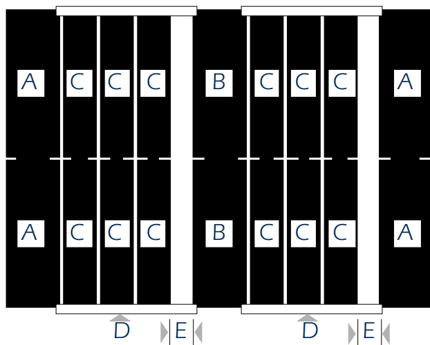
Voorbeeld 2: Dubbel verrijdbaar stellingstelsysteem met uitwendige geleiders (max. diepte 3100 mm)
